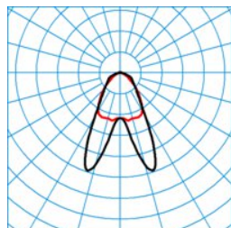
ELINE LDAN40-110 ML 830 L150 4 20 ■ C0 - C180
