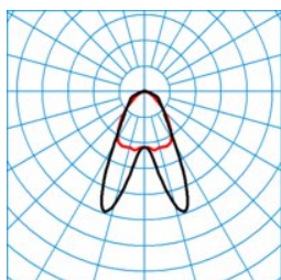
ELINE LDAN40-110 ML 830 L150 0 20 ■ C0 - C180
