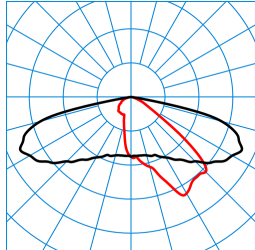
LIQ 50N-AB2L-LR-SLR2/6800-740 6G1 ET (CLO end value) TX777204
