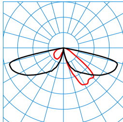
CS 19 100-AB2L-LR/3800-730 4G1S ET (CLO end value) TX300026
