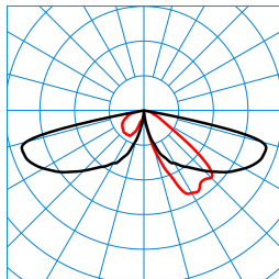
CS 19 100-AB2L-LR/3800-730 4G1S ET (CLO initial value) TX300027
