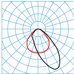
Luceos D/H2-L CDP-A 6500-840 ETDD 01 (Ceiling D2 ZD/01+EB3) TX277137
