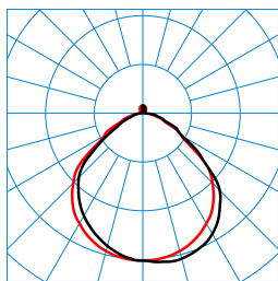
Luceos D/H2-L CDP-A 6500-840 ETDD 01 (Pendant ZS/ZST+EB3) TX245965
