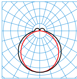
Olisq LWD3 DW 75-840 ET2 IP54 IK TX564630
