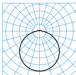
Olisq RWD3 DW 30-840 ETBLE +CAS-S + Olisq RWD3 ZDR 1/2 03 TX565806
