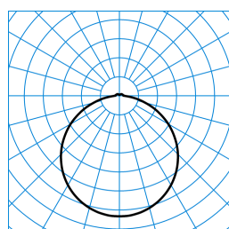
Olisq Act RWD4 DW 40 ETDD8 PC + Olisq RWD4 ZDR 1/2 01 (ActDWW) TX427238 ■ C0 - C180 ■ C90 - C270
