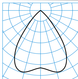
InperiaL G2 C07 BR19 1800-830 ET 03 ■ C0 - C180 TX768190
