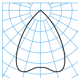
InperiaL G2 C07 BR19 1800-830 03 + DA 03 ■ C0 - C180 TX052823
