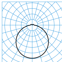
Olisq RWD3 DW 50-840 ETDD IP54 + Olisq RWD3 ZDR 1/2 03 TX42685
