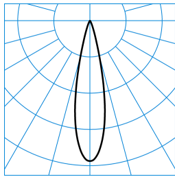
7651 LentyP L-SP 40-EC M39 ETBLE 03 (150) TX782412
