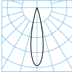
7651 LentyP L-SP 40-EC M39 ETBLE 03 (225) TX782413
