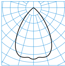
InperiaL G2 C07 BR25 4700-840 ETDD 03 ■ C0 - C180 TX769261
