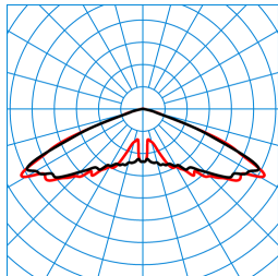
Publisca P1W-RB6L-LRA/1200-730 2G1S ET (CLO initial value) TX300768
