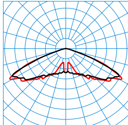
Publisca P1W-RB6L-LRA/1200-730 2G1S ET (CLO end value) TX301170
