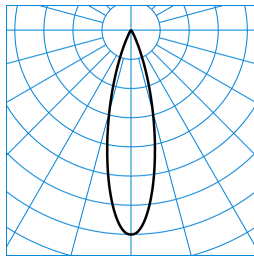
7651 LentyP L-MF 30-BF M54 ETDD 05 (150) TX782111
