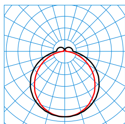
Olisq Act LWD3 DW 30 ETDD8 IP54 IK (ACTDCW) TX430126
