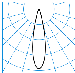
7651 LentyP L-SP 40-EW M48 ET 03 (225) TX782443
