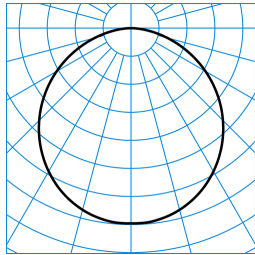
Olisq RWD2 DW 40-840 ET HFS + Olisq RWD2 ZDR 1/1 01 TX425972
