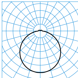
Olisq RWD2 DW 20-830 ETBLE +CAS-S IP54 + Olisq RWD2 ZDR 1/2 03 TX565950
