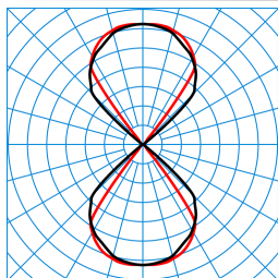
Skeo Q-W1-DI GT RB9R-RB9R/180-830 ET TX773819
