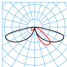
LTX LT-AB2L-LRA/15/18/26-740 4G1 (1800 lm) TX084098
