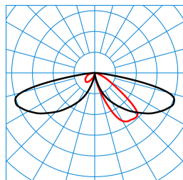
LTX LT-AB2L-LRA/15/18/26-740 4G1 (2600 lm) TX084099
