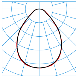
ArimoFit G2 M59 PW19-X 53-840 ETDD + ArimoFit G2 Sky M59-TS ZER TX426838
