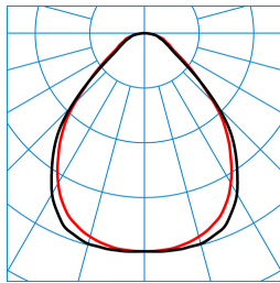
ArimoFit G2 M59 PW19-X 53-840 ETDD TX376420
