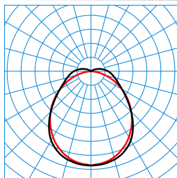
OleveonF 15 L 6000-840 ETDD PC+LLWC LV TX719543
