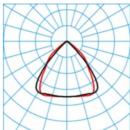
ELINE HE LW2260-160 ML 830 L225 4 20 ■ C0 - C180
