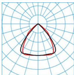
ELINE HE LW2260-160 ML 830 L225 2 20 ■ C0 - C180
