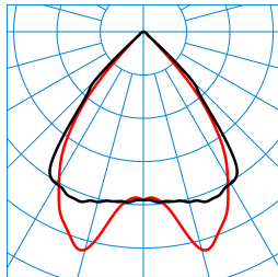
SFlow C2-L MRX LED4000-840 ET 01 TX721255
