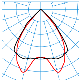
SFlow C2-L MRX LED4000-840 ET 01 TX771628
