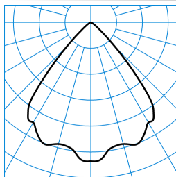
InperlaLP C05 HR22 IP 1800-830 ET 03 TX771330
