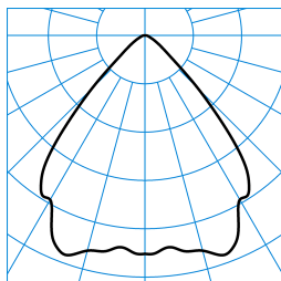
InperlaLP C05 HR22 IP 1800-830 03 + DA 03 TX052455
