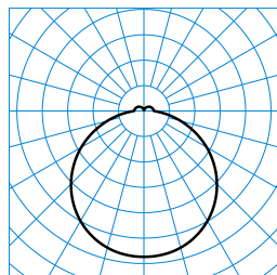
Olisq RWD1 DW 20-840 ETDD + Olisq RWD1 ZDR 1/2 03 TX425806
