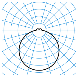
Olisq RWD2 DW 14-40/4/ML-830 PC ET (stage 1) TX776060
