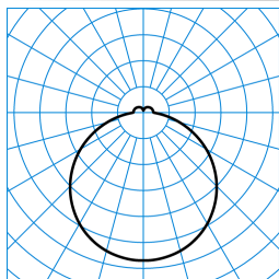
Olisq RWD2 DW 14-40/4/ML-830 PC ET (stage 0) TX776059
