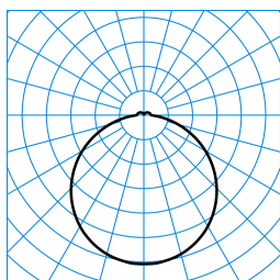
Olisq RWD2 DW 14-40/4/ML-830 PC ET + Olisq RWD2 ZDR 1/2 01 (stage 0) TX776079
