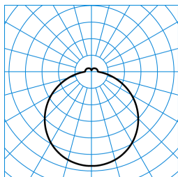
Olisq RWD2 DW 14-40/4/ML-830 PC ET (stage 2) TX776061
