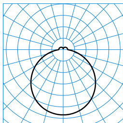
Olisq RWD2 DW 14-40/4/ML-830 PC ET (stage 3) TX776062
