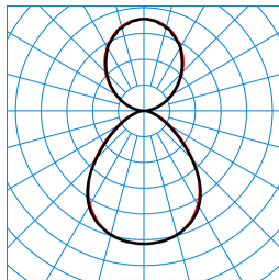
Lunexo H1 CDP-I 6500 830 ETDD +LLWS 01 TX773808
