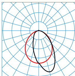
SFlow C2-L MLA LED4600-830 ETDD 01 TX721357
