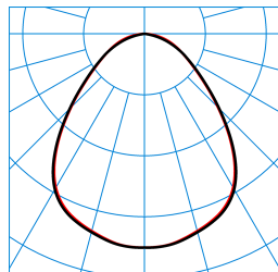
7651IP MironaF B 130-840ET L150 01 (LEO2) TX306248
