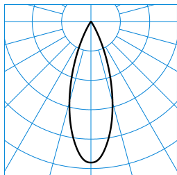
7651 LentyP L-FL 40-840 M35 ETBLE 01 (225) TX776118
