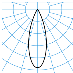
7651 LentyP L-FL 40-840 M35 ETBLE 01 (150) TX776117
