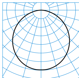
Olisq RWD2 DW 40-830 ET IP54 PC + Olisq RWD2 ZDR 1/1 01 TX425949
