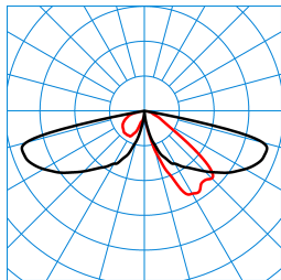
CS 19 100-AB2L-LR/4600-730 4G1S ET (CLO initial value) TX300031
