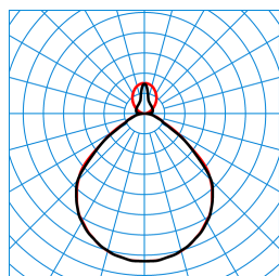
Luceos D/H2-L CDP 8400-840 ETDD 01 (Ceiling D2 ZD/03+EB3) TX547714
