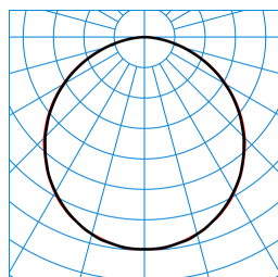
Olisq QWD2 DW 20-830 ETBLE +DMR IP54 IK + Olisq QWD2 ZDR 1/1 01 TX461931
