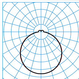
Olisq QWD2 DW 20-830 ETBLE +DMR IP54 IK TX777354
