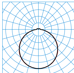
Olisq QWD2 DW 20-830 ETBLE +DMR IP54 IK + Olisq QWD2 ZDR 1/2 01 TX462180
