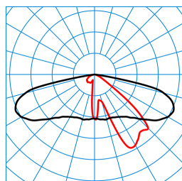
Publisca P1-AB2L-LRA/1200-740 2G1S ET (CLO initial value) TX300717
