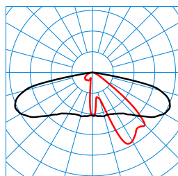
Publisca P1-AB2L-LRA/1200-740 2G1S ET (CLO end value) TX301535
