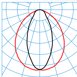
Nextrema G3 TB 60-840 ET +LV TWP TX768233
