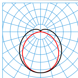
Tugra 15 PL 50-840 ETDD EB3 23 TX778246
