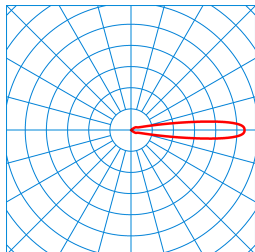
CS 19 S-MOD RE6R-LR/3200-740 1G1 ET (CLO initial value) TX369172
