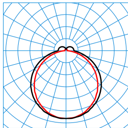
Olisq LWD2 DW 60-840 ET HFS IP54 TX375437
