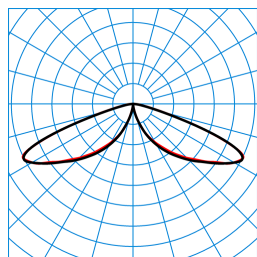
LTX ZT-RB6L-LRA/15/18/26-740 4G1 (1800 lm) TX084227
