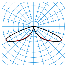
LTX ZT-RB6L-LRA/15/18/26-740 4G1 (1500 lm) TX084226
