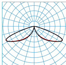
LTX ZT-RB6L-LRA/15/18/26-740 4G1 (2600 lm) TX084228
