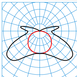
AragF 15 PXW 48-840 ETDD +LLWC LV PC TX769289
