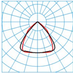
ELINE HE LW2260-160 ML 840 L225 0 50 ■ C0 - C180
