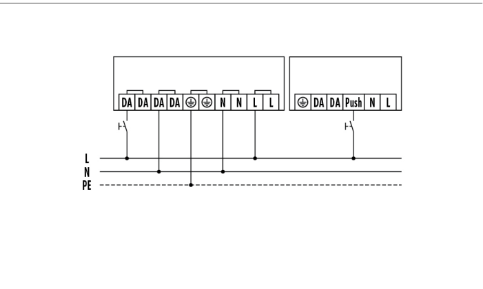
Standaardschema met optionele functie SwitchDIM (PushDIM).
