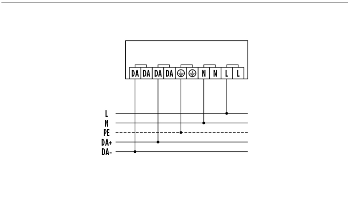
Standaardschema DALI/DALI-2.
