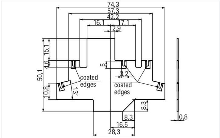
PCB dimensions
