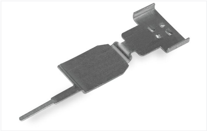
Shield termination WINSTA® MINI 5-pole
