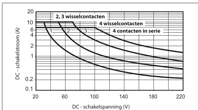
H 58 - Gelijkstroomvermogen bij DC1 - Belasting
