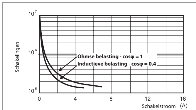
F 58 - Elektrische levensduur bij AC 4 wisselcontacten
