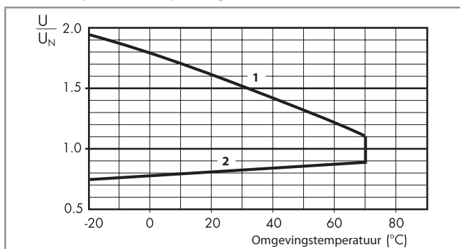
R 58 - DC-spoelen-werkspanningsbereik
