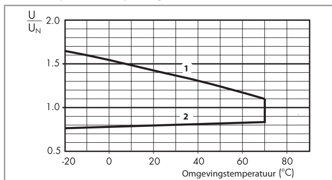
R 58 - AC-spoelen-werkspanningsbereik
