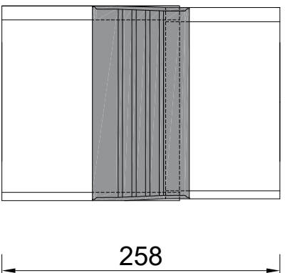
Bovenaanzicht Expansie-element
