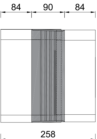
Bovenaanzicht Expansie-element
