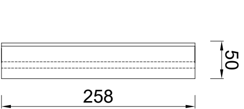
Bovenaanzicht kraalstuk
