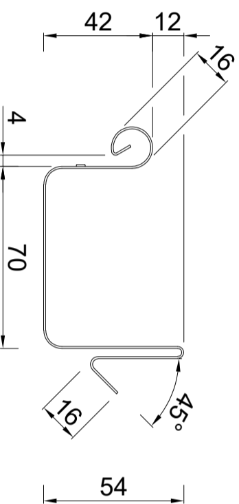
Balkon-klikgoot Doorsnede 3000x 0,70mm Artikelnummer: 0850001000
