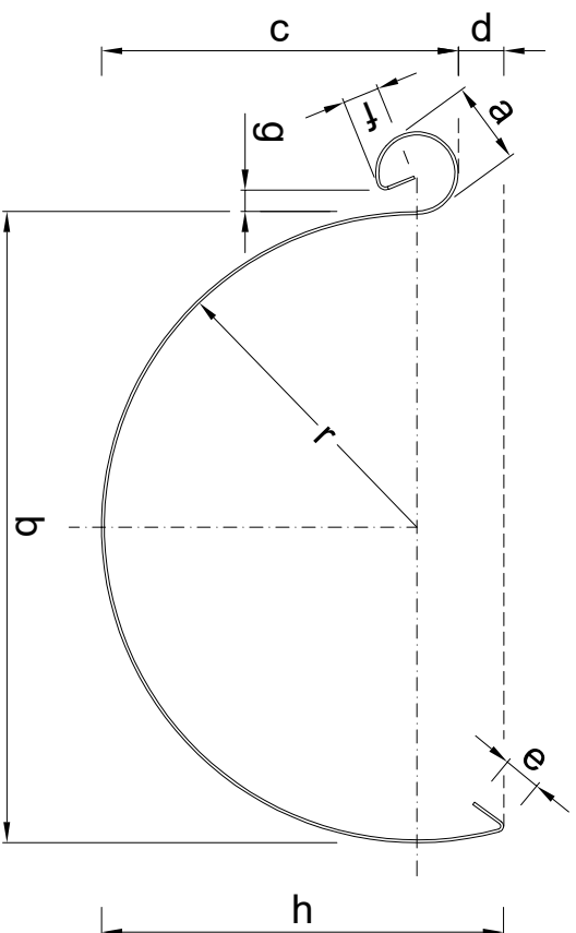
Doorsnede
